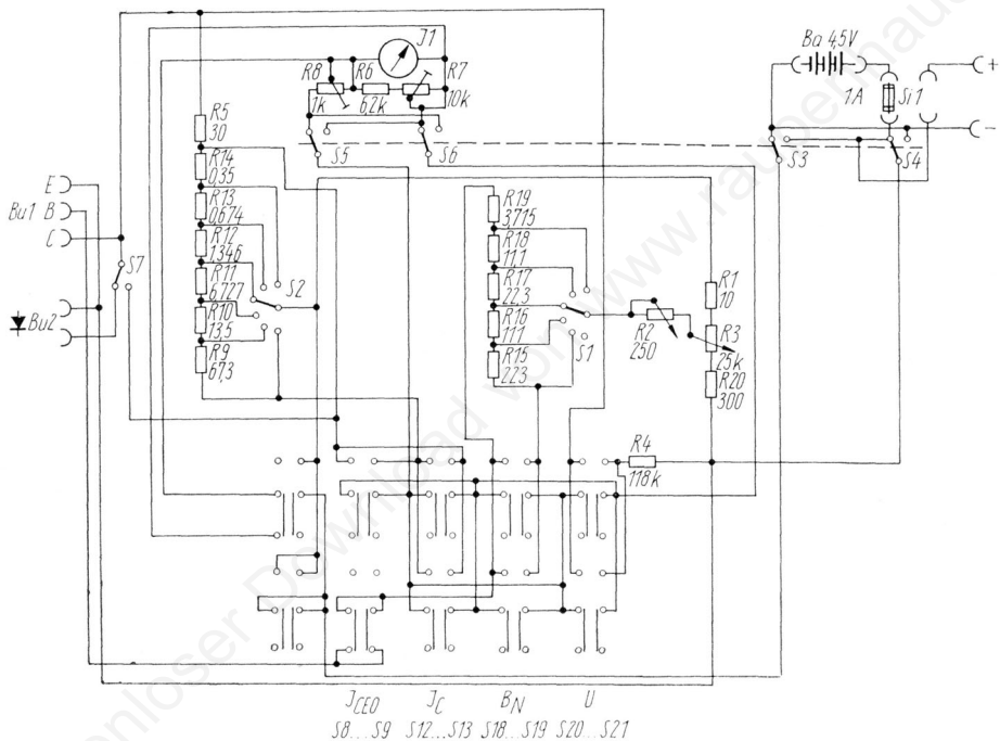
Transistoren-Prüfgerät Typ 1020a
